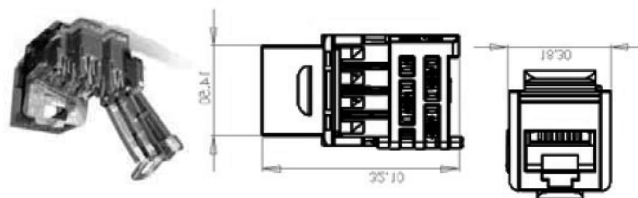
Connettore di tipo RJ45 Keystone Jack non schermato
